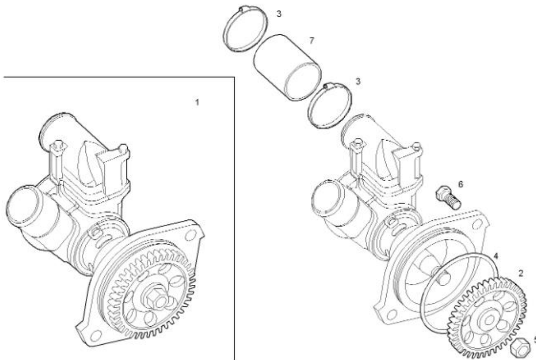
Vue éclatée pompe
