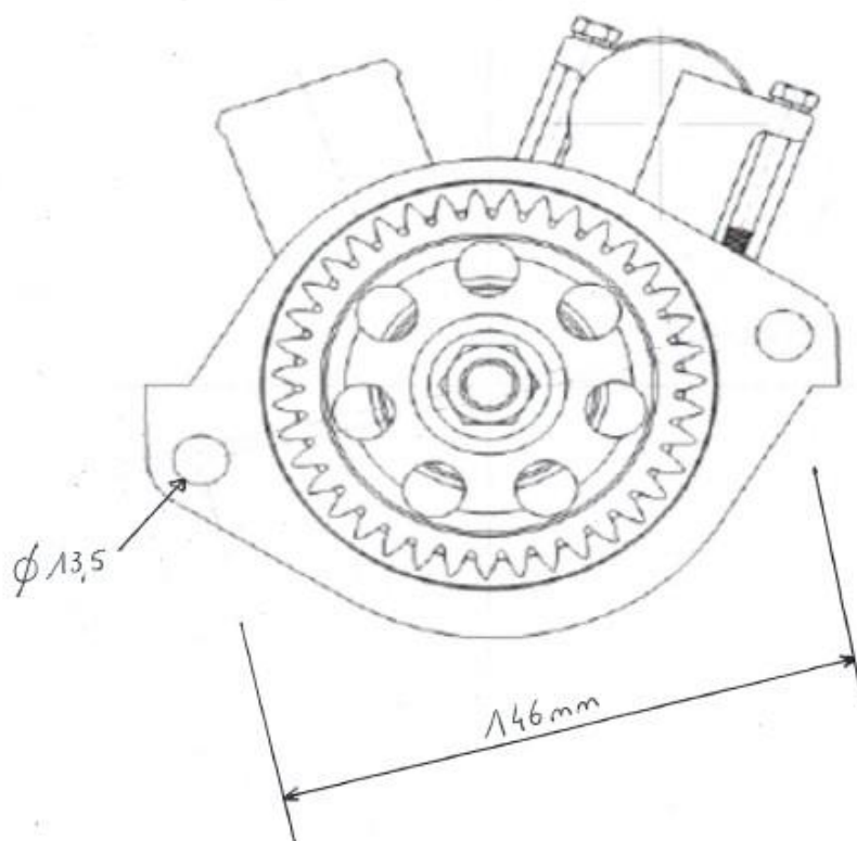
Montage pompe
