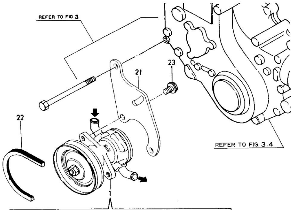
Fig. 33 冷却水ポンプ(海水) COOLING SEA WATER PUMP
