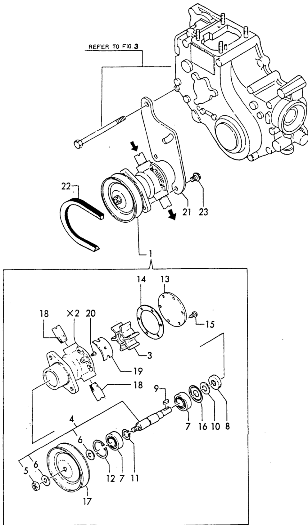
Fig. 33 カイスイポンプ COOLING SEA WATER PUMP
